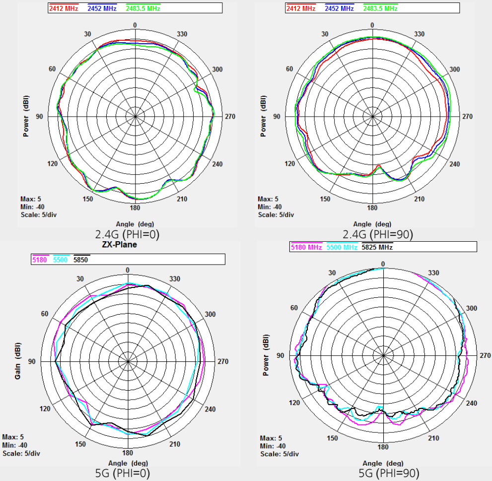
AP4050DN 天线方向性图
